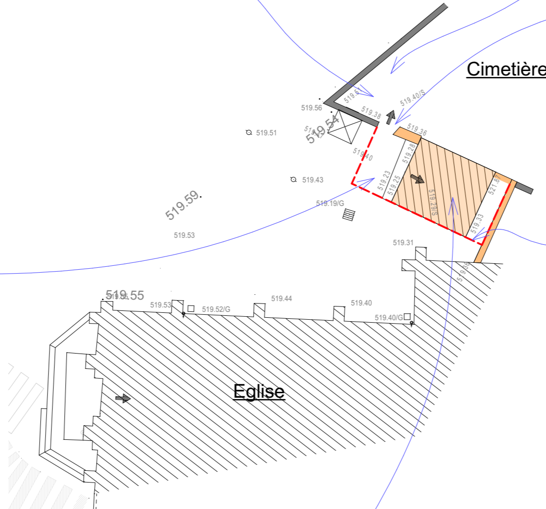
1.2.5.6 - Démolition du dallage et de la rampe
